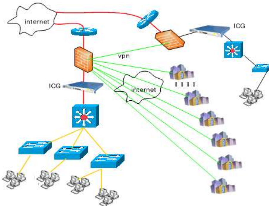
图 6：长城润滑油公司互联网访问管理方案部署拓扑示意图
